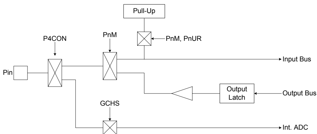
图 10-1. I/O 口电路简图
