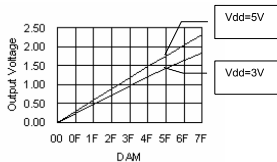
图 12-3. DAC 输出电压 ( V_{dd}=5V / 3V )
