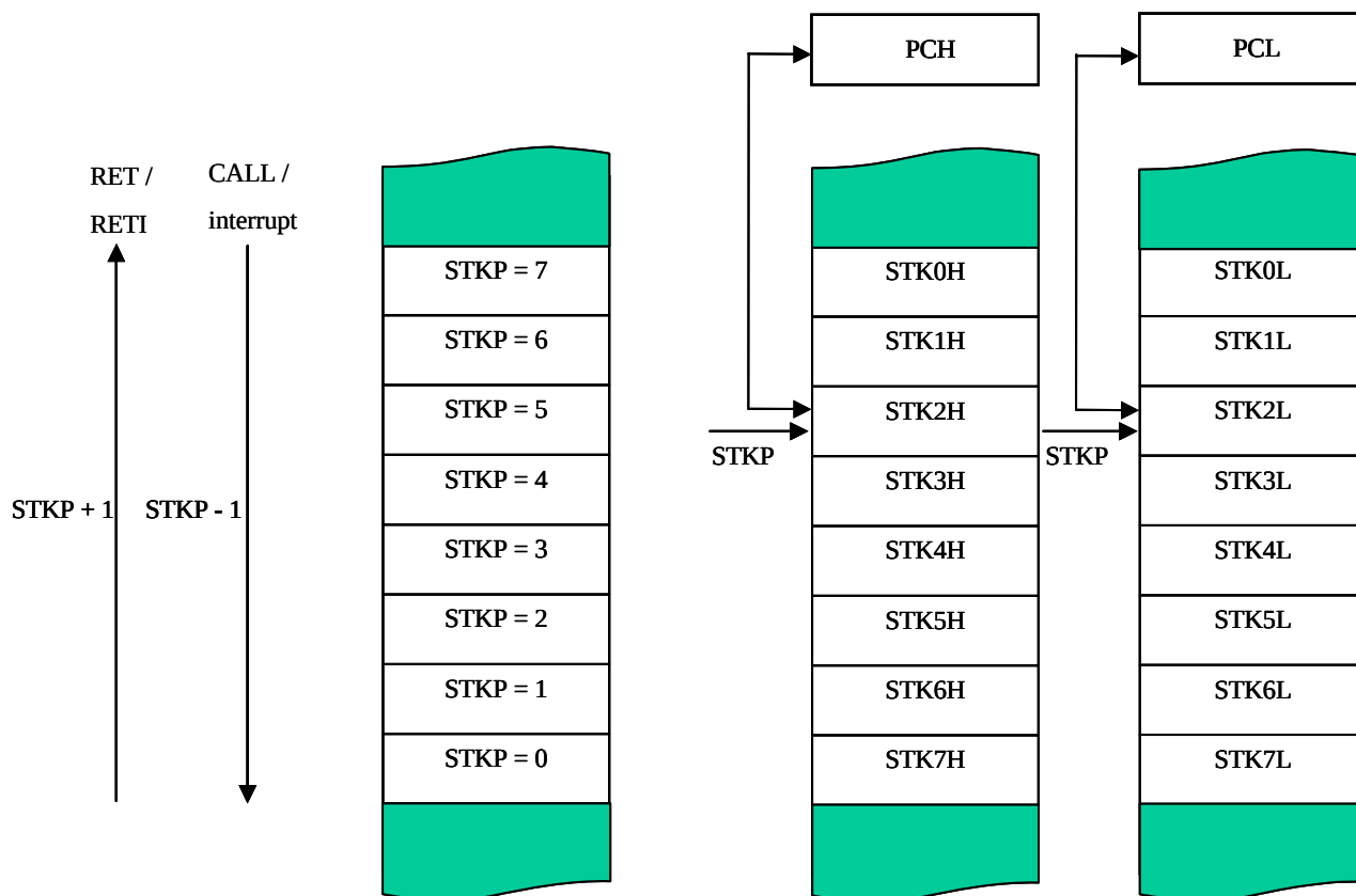
图 3-3 堆栈
