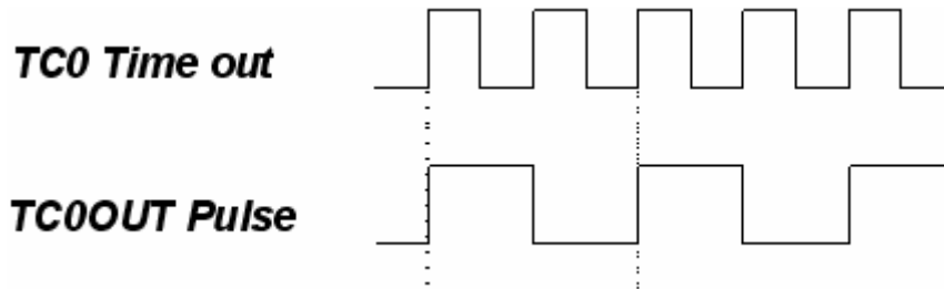
图 8-2 TC0OUT 频率图
