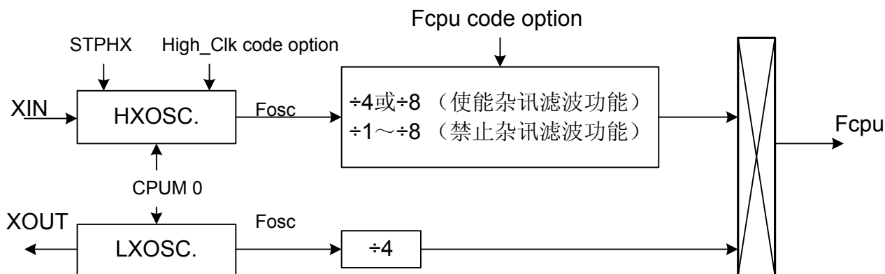
图 7-1 系统时钟框图
