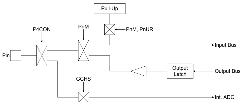
图 1-1. 引脚电路结构图
